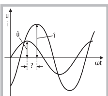
Puissance réactive
